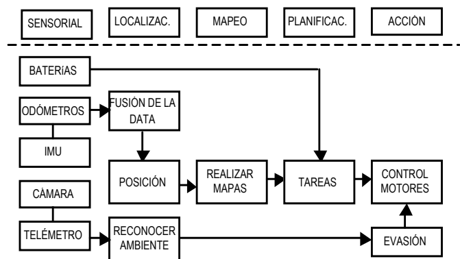
Figura 2. Diagrama de la Arquitectura de software seleccionada para la plataforma robótica.
